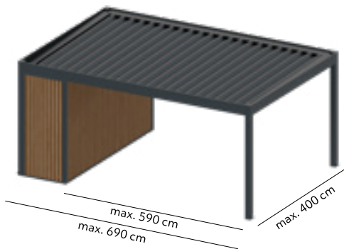
Einzelcarport | One-station Carport | Carport à station unique
