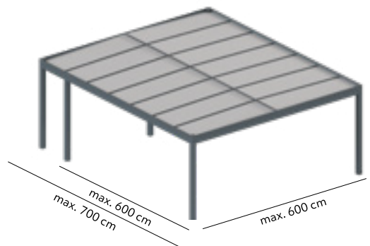
Zweifach geneigten Dach | Double-pitched roof | Toit à deux pentes
