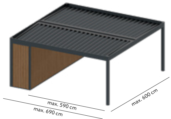
Doppelcarport | Two-stations Carport | Carport à deux stations
