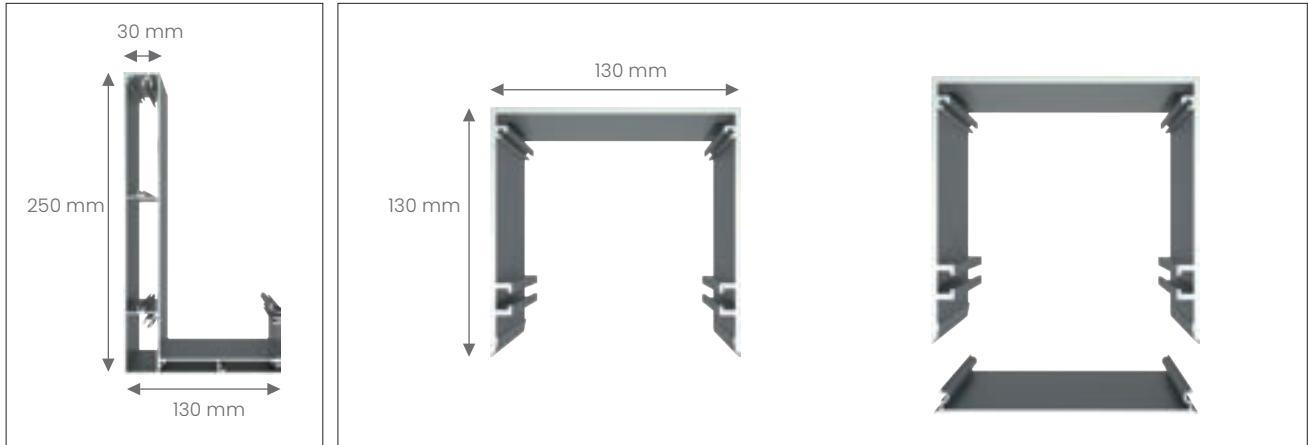
Durschnitt des Konstruktionsprofils Construction profile
